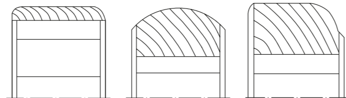
1 Inserto encolado 2 Reborde encolado abombado 3 Reborde encolado softline
